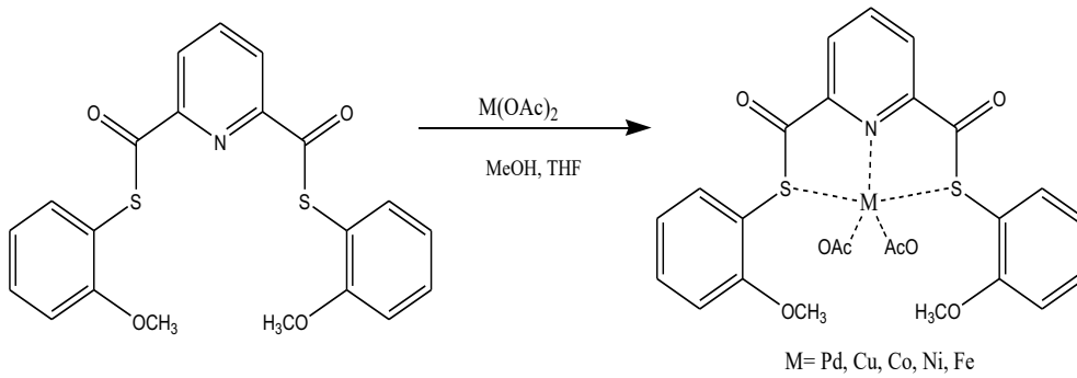
Şekil1. Tiyoeater Ligandının Sentezi
