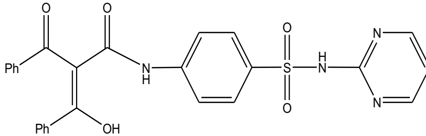
Şekil1. N-karboksamit ligandın Yapısı
